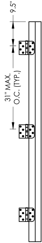
HINGE JAMB
